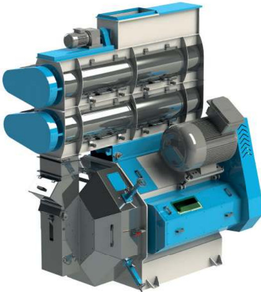
PELET PRESİ PELLET MILLS PRESSE PELLETT ПРЕСС-ГРАНУЛЯТОР مكبس الحبيبات
